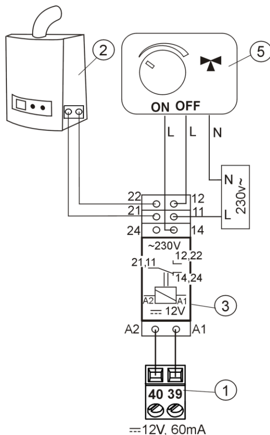
Электрическая схема подключения управления переключающим клапаном резервного котла, где: 1 – регулятор, 2 – резервный котёл, 3 – реле, 5 – привод переключающего клапана (с ограничительными выключателями), Внимание: зажимы 22,21,24 должны быть гальванически отделены от зажимов 12,11,14.
